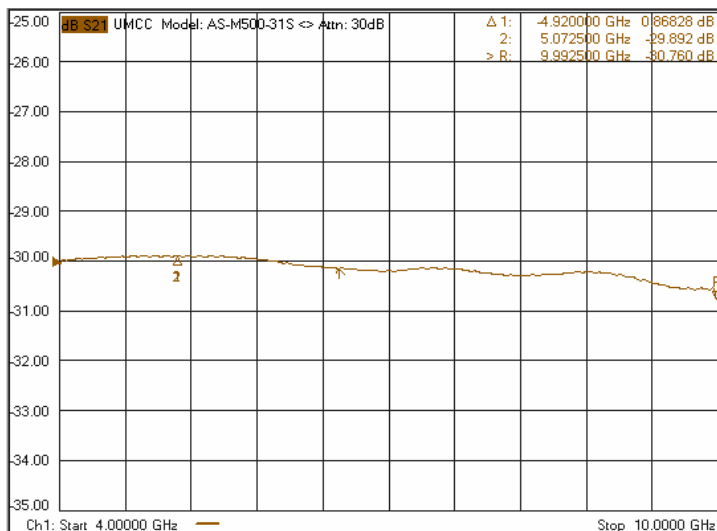
-Attenuation 30dB
