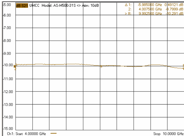
-Attenuation 10dB
