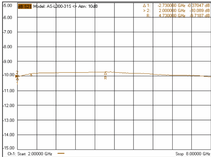
-Attenuation 10dB
