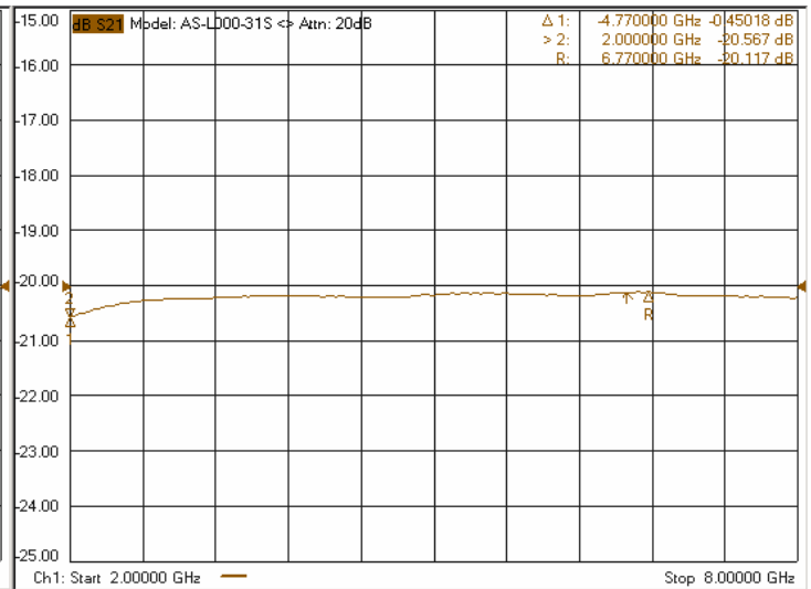
-Attenuation 20dB
