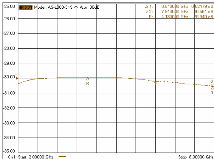
-Attenuation 30dB
