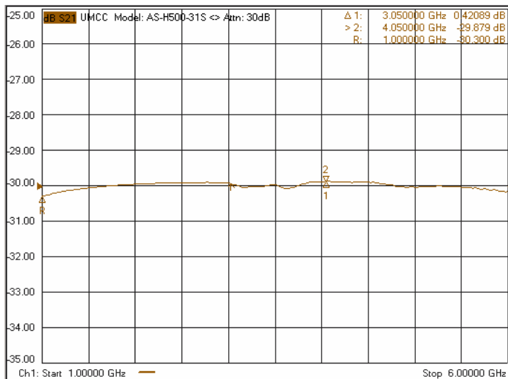
-Attenuation 30dB
