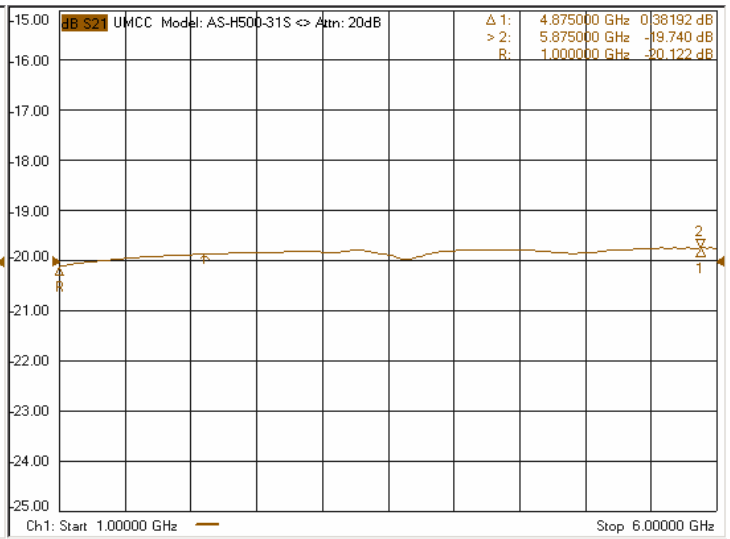
-Attenuation 20dB
