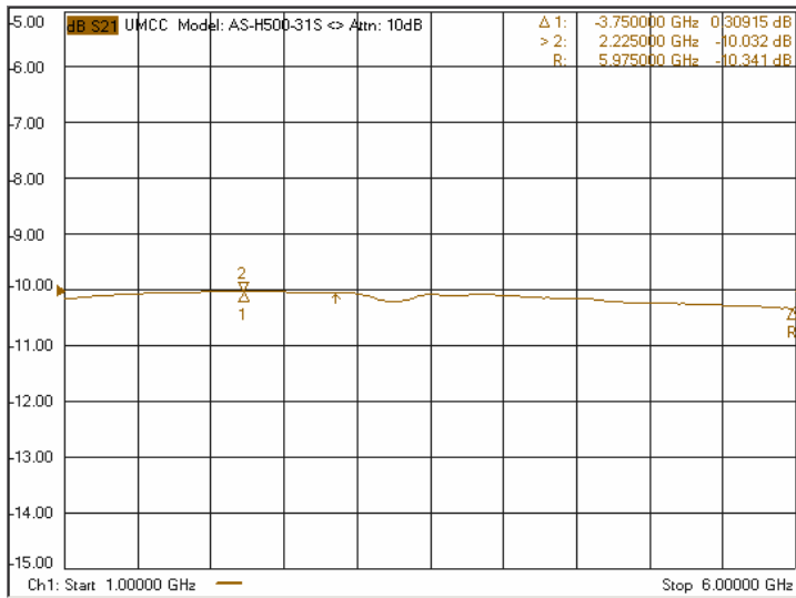
-Attenuation 10dB
