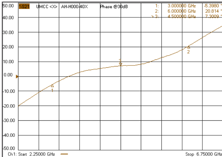
Phase Shift @ 30dB Attn.
