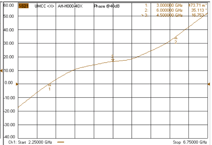
Phase Shift @ 40dB Attn.
