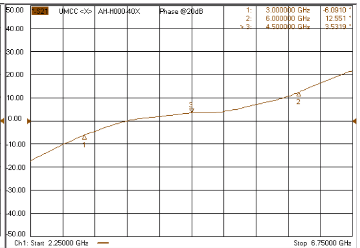
Phase Shift @ 20dB Attn.
