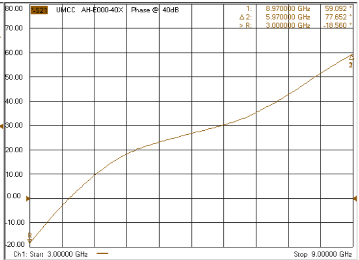
Phase Shift @ 40dB Attn.
