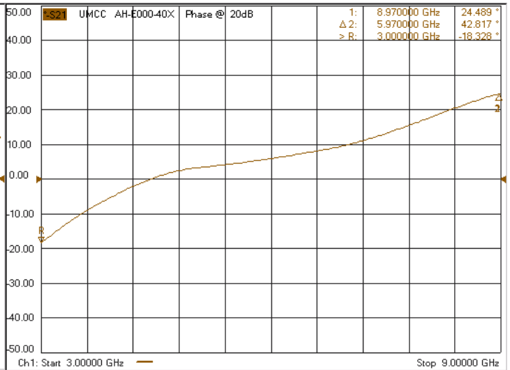
Phase Shift @ 20dB Attn.
